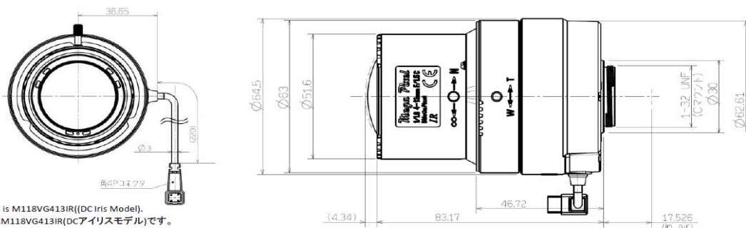
Drawing 外観図面
